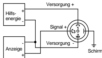
Dreileiterschaltung
