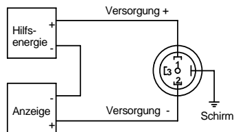
Zweileiterschaltung
